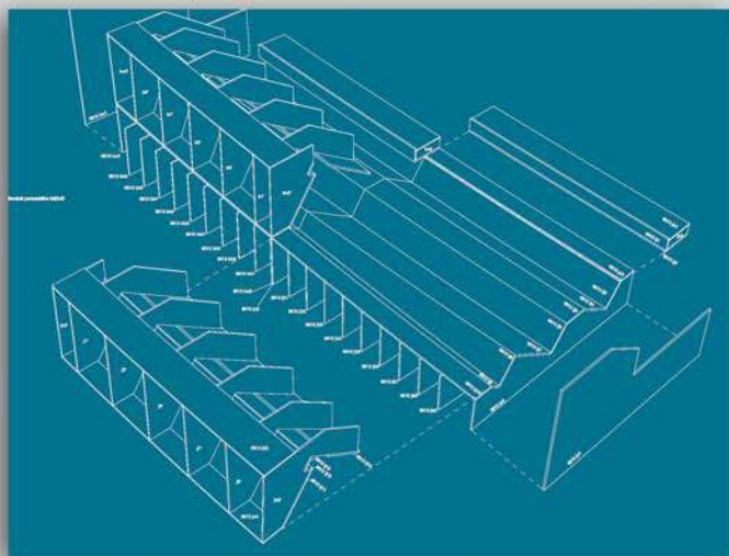
FASABLONOK KIMARÁSA HOLZER 7013 TÍPUSÚ CNC MEGMUNKÁLÓVAL
